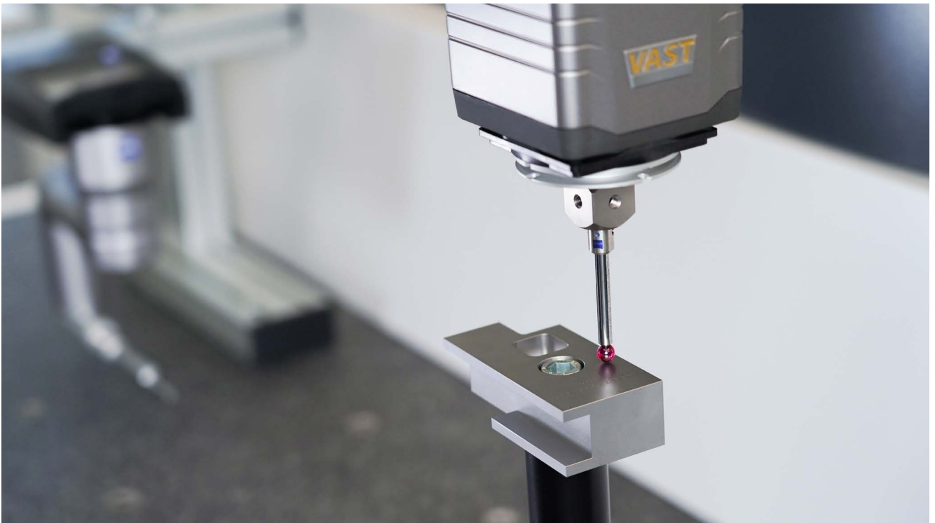
ZEISS Koordinatenmessgerät mit installiertem ZEISS Smart Services Remote Health Check Kit, vorbereitet für den Health Check.
